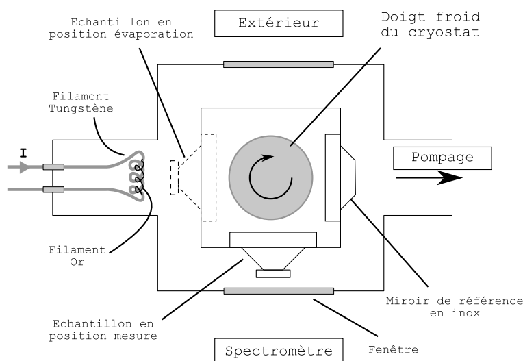
FIGURE 5.6 – Dispositif d'évaporation d'or in-situ . Un petit filament en or est enroulé sur un autre filament de tungstène, en faisant passer un courant électrique dans le filament de tungstène, on sublime l'or qui s'évapore et se dépose sur l'échantillon.
