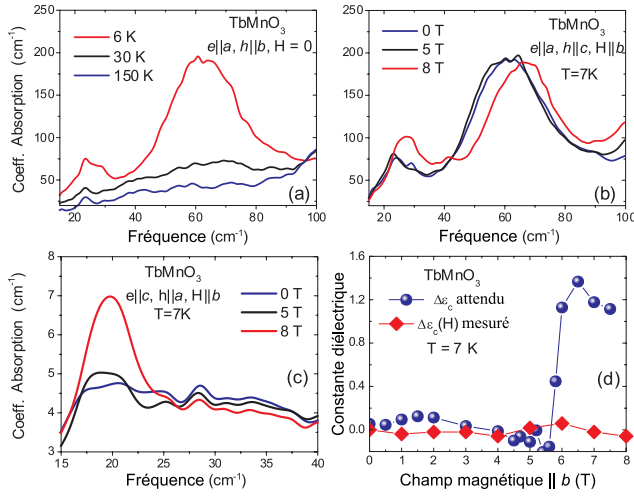
FIGURE 3.6 – Electromagnons de TbMnO 3 mesurés par spectroscopie infrarouge par Valdés Aguilár et al. (2009) . (a) Dépendance en température du coefficient d'absorption montrant les deux pics d'électromagnons à 20 et 60 cm -1 en dessous de T_N . (b) Dépendance en champ magnétique du spectre d'absorption à basse température, dans la phase de fort champ magnétique, la fréquence des électromagnons augmente légèrement mais ils restent dans la direction a . (c) Excitation apparaissant sous fort champ magnétique, cette excitation d'origine magnétique car sa contribution attendue à la constante diélectrique n'apparaît pas dans les mesures statiques (d)
