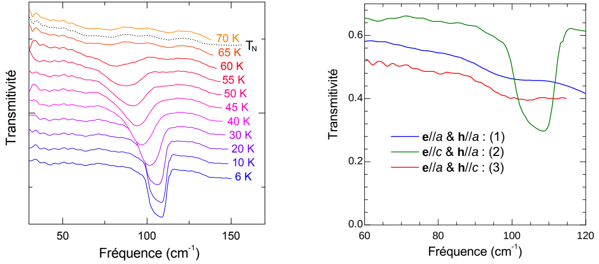
FIGURE 7.15 – Transmittivité de \text{MnF}_2 dans l’infrarouge lointain montrant le pic d’absorption du double-magnon. À gauche : évolution du pic d’absorption en fonction de la température mesuré dans la configuration (2) sur un échantillon de 0.4 mm d’épaisseur. À droite : mise en évidence de la règle de sélection liée au champ électrique de la lumière : le double magnon est actif uniquement pour E \parallel c . Les nombres entre parenthèses indiquent la configuration de mesure (voir figure 7.11)
